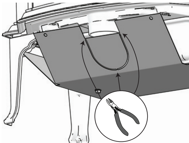
Fig. 7a Montare il collegamento di alimentazione dell'aria esterna
