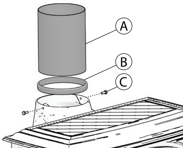
Fig. 5 Assemblare il condotto
