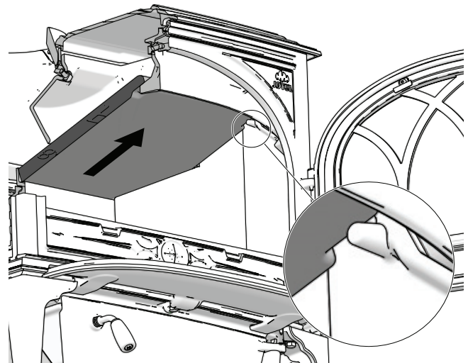
Fig. 15a Loosen the baffle plate
