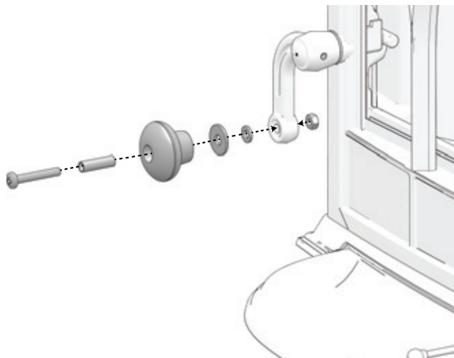
Fig. 3 Assemblare la maniglia del portello
