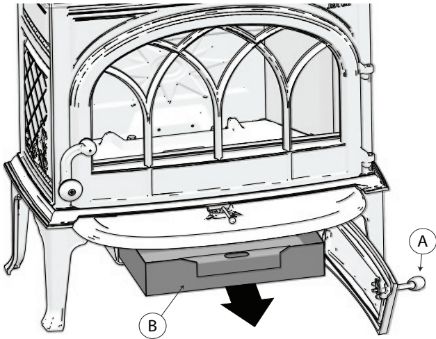
Fig. 13 Cassetto ceneraio
