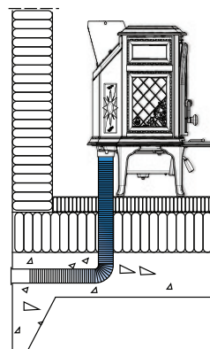
Fig.6b Attraverso il pavimento e la piastra di terra
