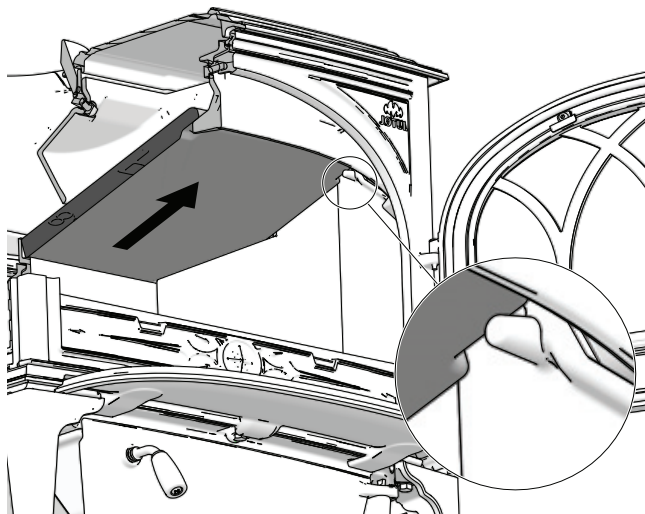
Fig. 15a Liberare la piastra del parafiamma
