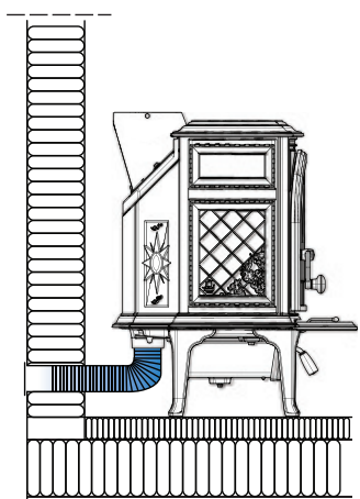
Fig.6a Attraverso una parete esterna
