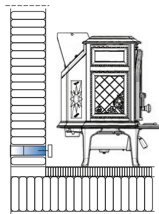
Fig.6d Indirettamente attraverso una parete esterna
