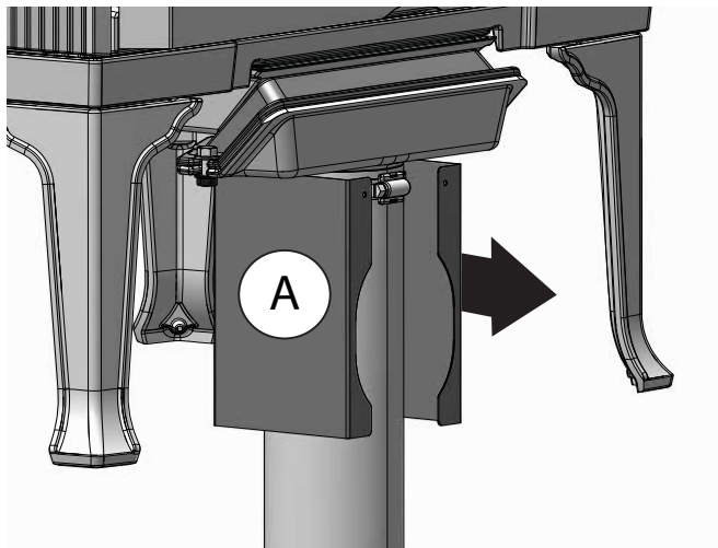
Fig. 8 Installazione del coperchio per aria esterna (Dotazione opzionale 50061978)
