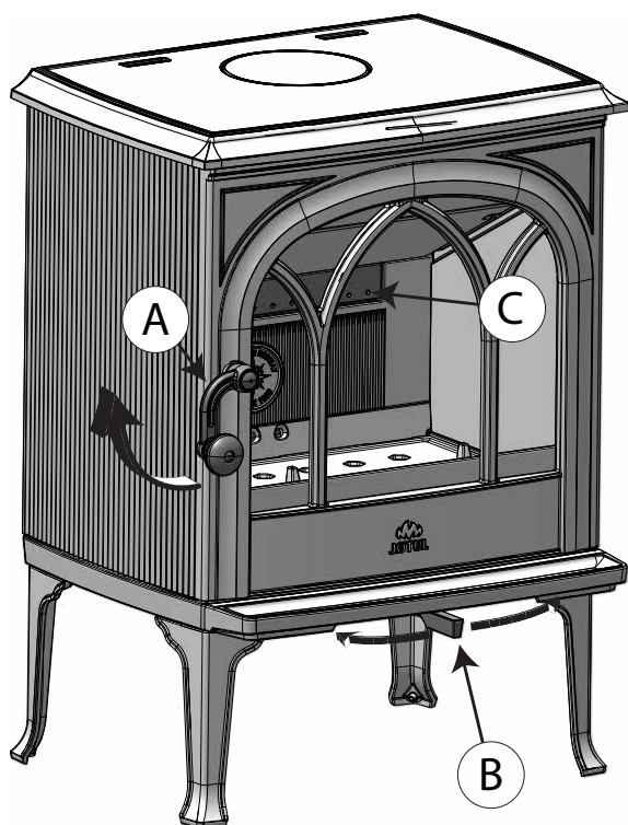
Fig. 10 Operating options on Jøtul F 200 V2 IT/F 205 V2 IT
