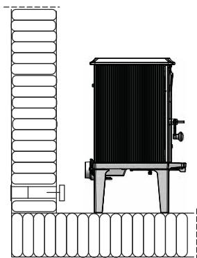
Fig. 5d indirettamente attraverso una parete esterna
