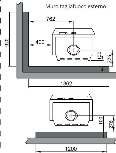
Muro tagliafuoco esterno
