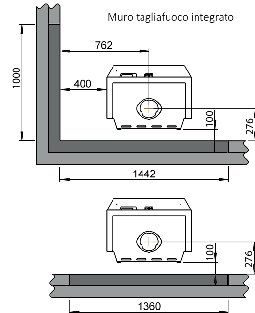
Muro tagliafuoco integrato
