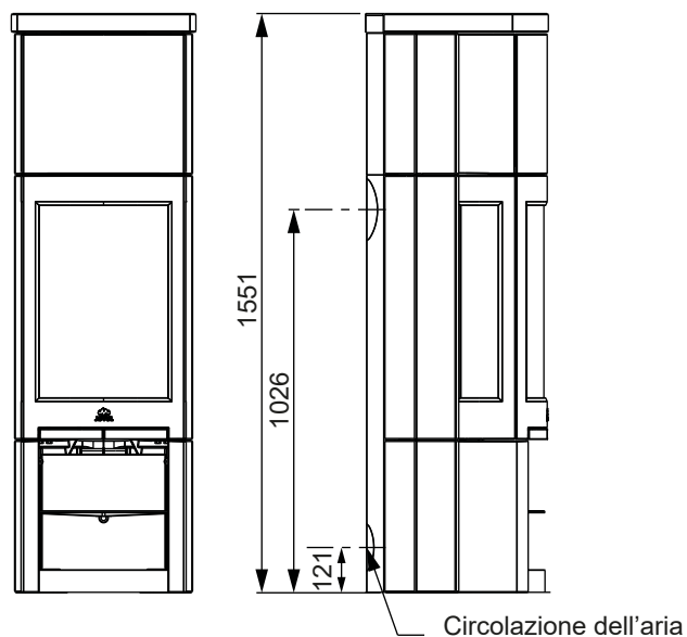
Jøtul F 377 Advance con High Top
